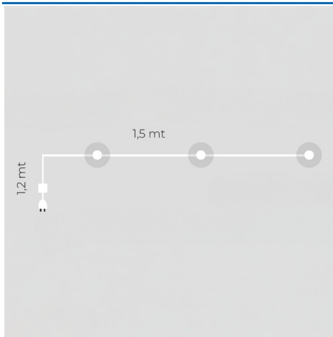
DOTS Stecker-Set Weiss für 3x E27 LED Lampen
