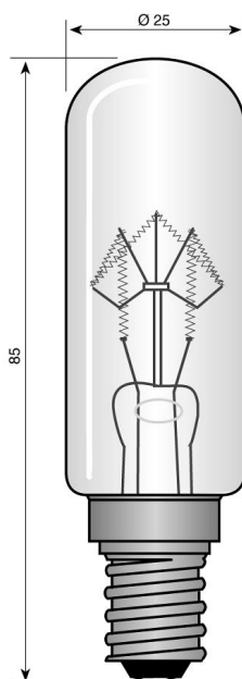
E14 25x 85 mm 130V 15W frosted
