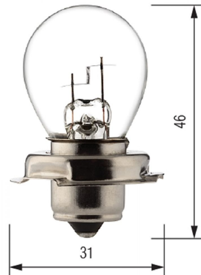
P26s 25.5x45 mm 12V 25W Motor
