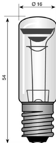
E14 16x54 mm 130V neon clear glass
