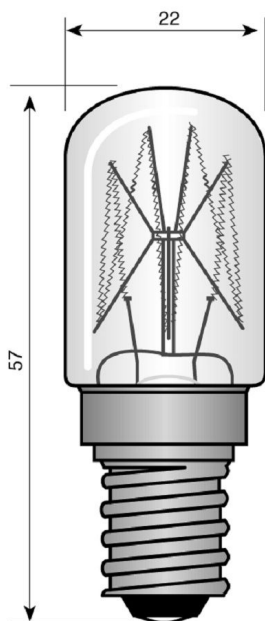
E14 22x57 mm 230V 25W clear
